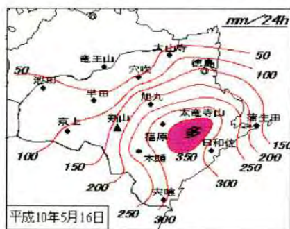
低気圧による大雨(ミリ)
