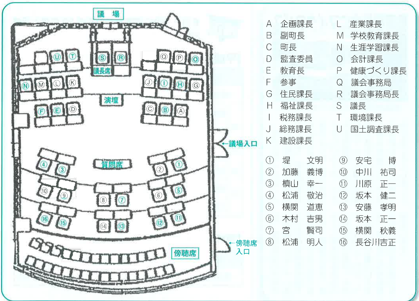
3階平面図 1/200
