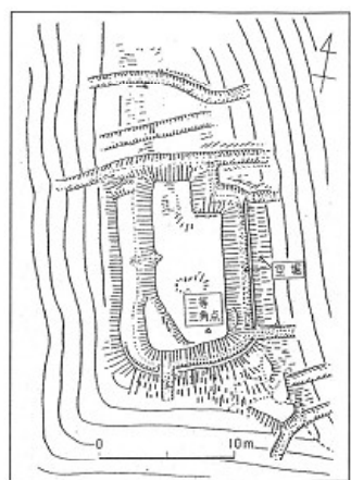
▲ 東山城跡 平面図
